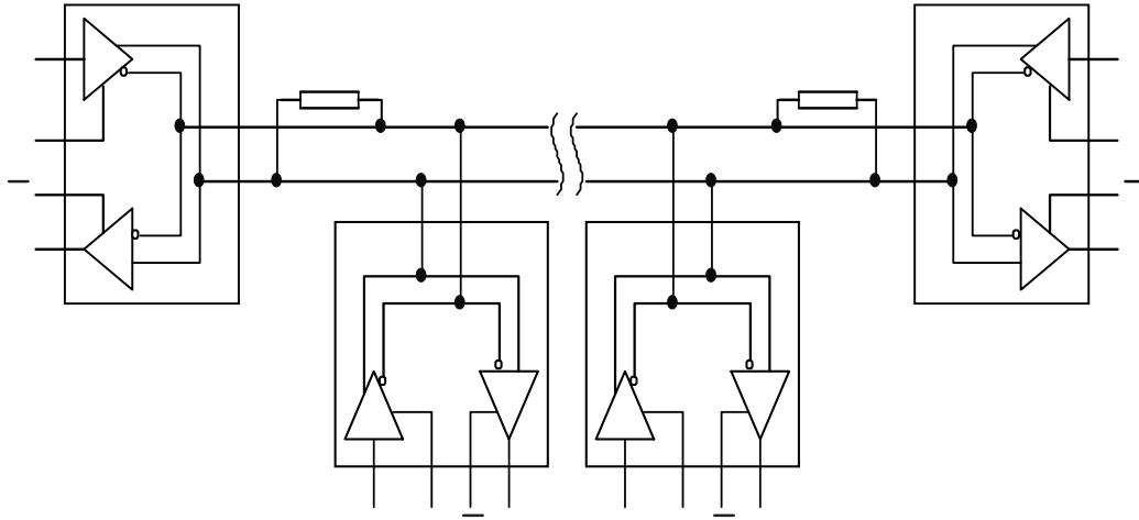
图 6 典型应用图
