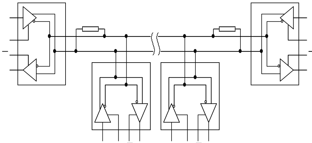
图 6 典型应用图
