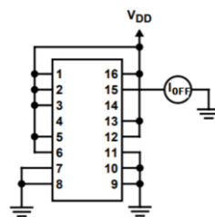
Fig. 3 所有通道关闭漏电流
