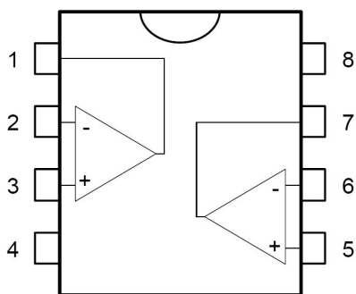
LM258(SOP8/DIP8/MSOP8/TSSOP8)
