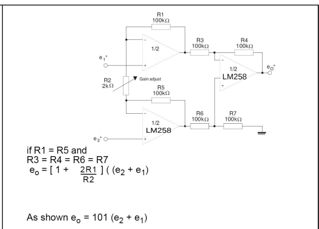
图6. 高输入阻抗可调增益直流仪表放大器
