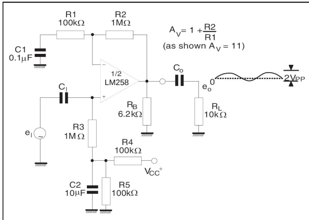
图3. 交流耦合正向放大器
