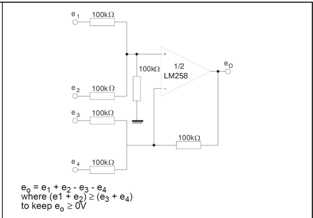
图4. 直流加法放大器
