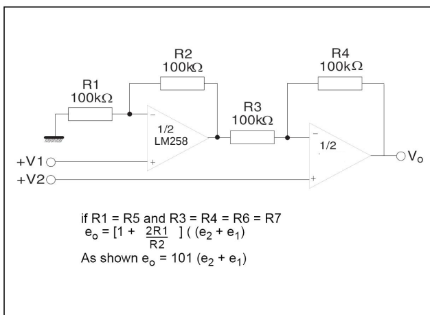
图5. 高输入阻抗,直流差分放大器
