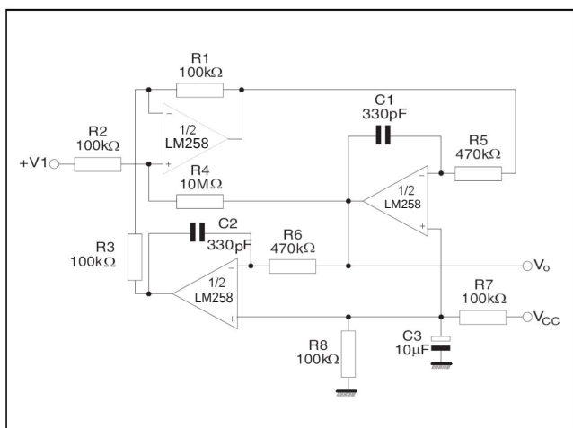
图9. 有源带通滤波器
