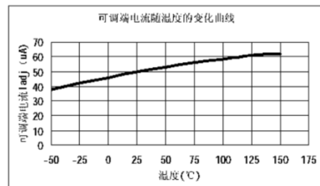
5. 可调端输出电流随温度变化曲线
