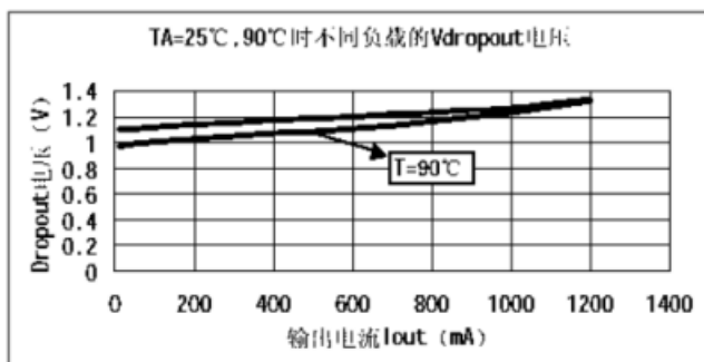
3. 负载特性曲线
