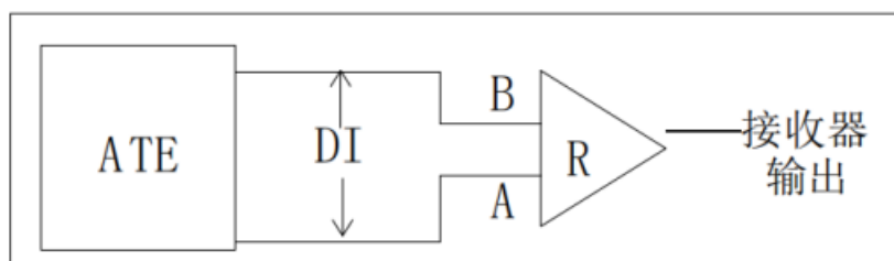
图 4 接收器传播延时测试电路
