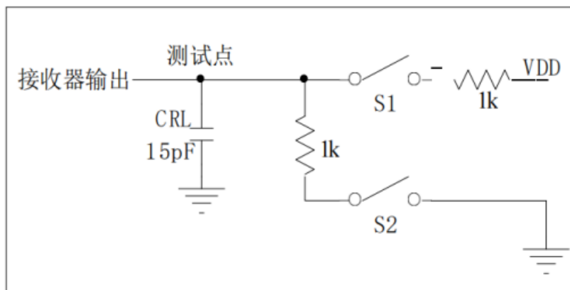
图 5 接收器使能/无效时序测试
