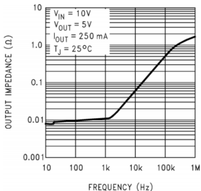
图 8 输出阻抗
