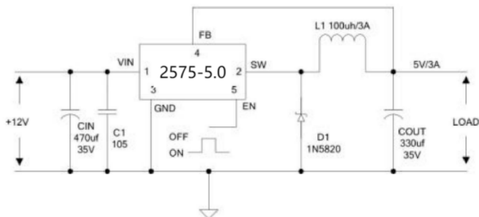
图6. 2575-5.0 系统参数测量电路
