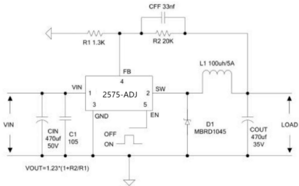
图 9. 2575-ADJ 大功率应用电路图 ( V_{IN}=24V, V_{OUT}=20V, I_{OUT}=2.5A )
