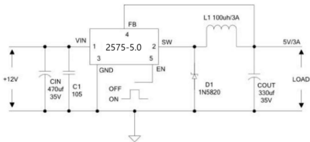
图4. 2575 系统参数测量电路(12V-5V/3A)
