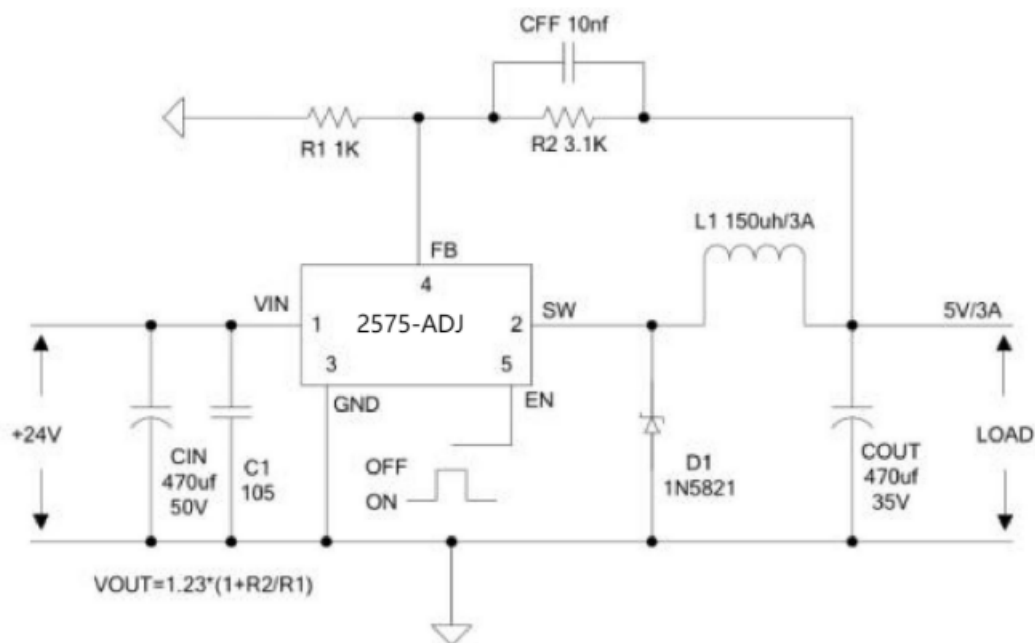
图 8. 2575-ADJ 系统参数测量电路
