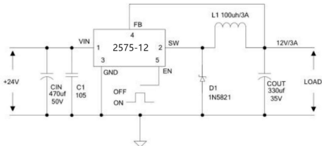
图 7. 2575-12 系统参数测量电路
