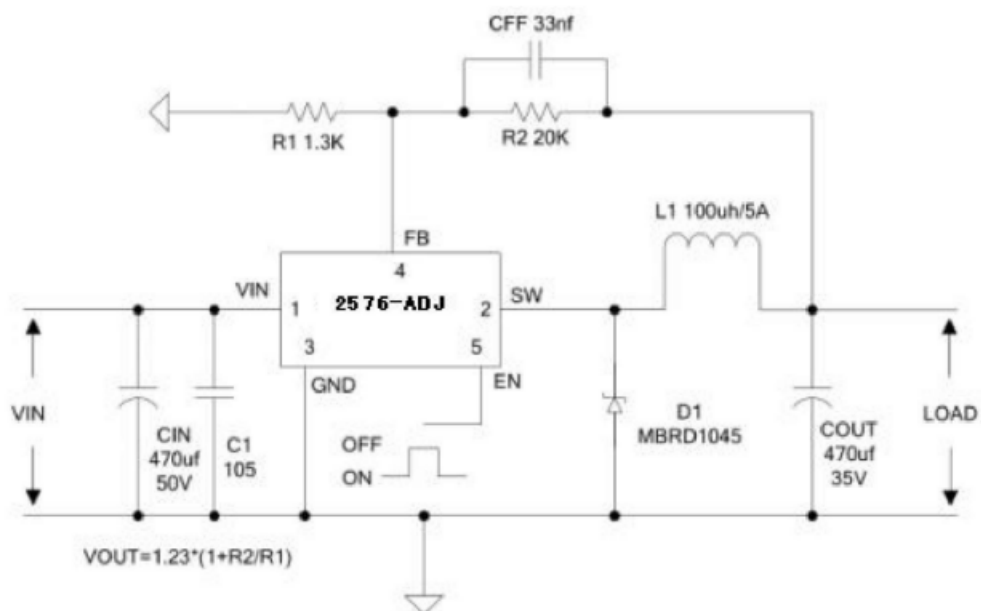
图 9. 2576-ADJ 大功率应用电路图 ( V_{IN}=24V, V_{OUT}=20V, I_{OUT}=2.5A )
