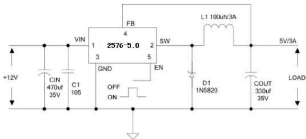
图4. 2576 系统参数测量电路(12V-5V/3A)
