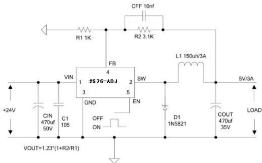
图 8. 2576-ADJ 系统参数测量电路
