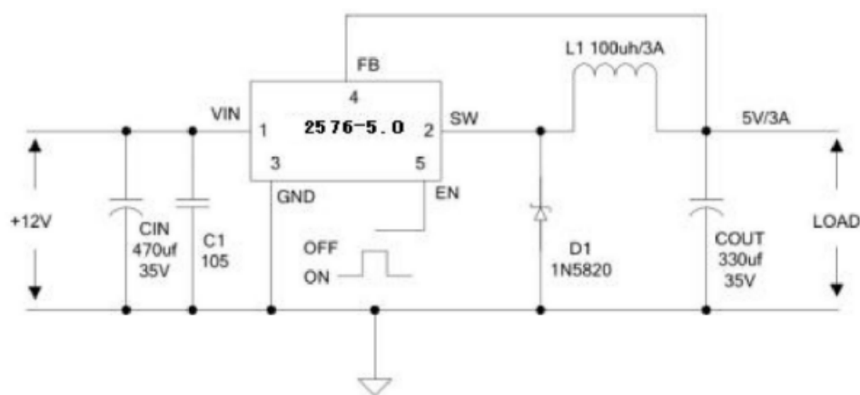
图6. 2576-5.0 系统参数测量电路
