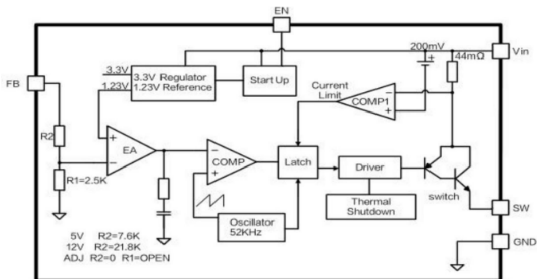
图3. 2576 方框图
