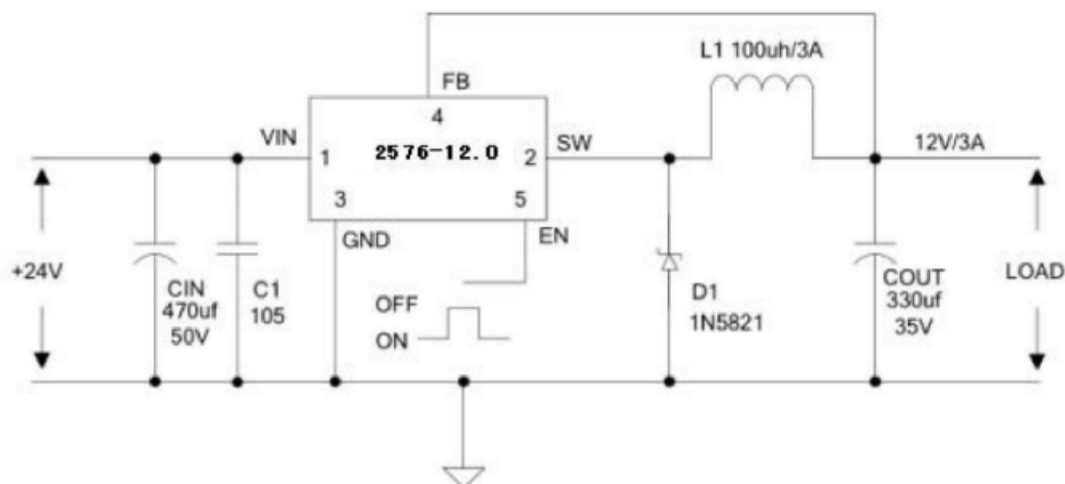
图 7. 2576-12 系统参数测量电路
