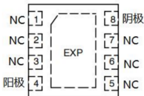
图 5 DFN-8 引脚图
