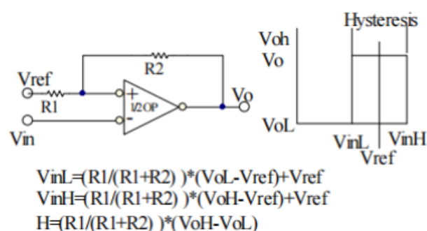
迟滞比较器
