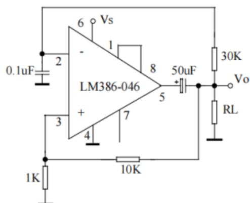
图6 方波振荡器
