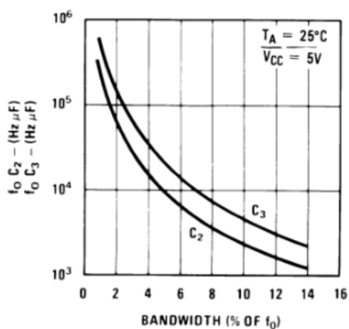
检测带宽随C2和C3的变化关系
