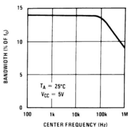
最大检测带宽
