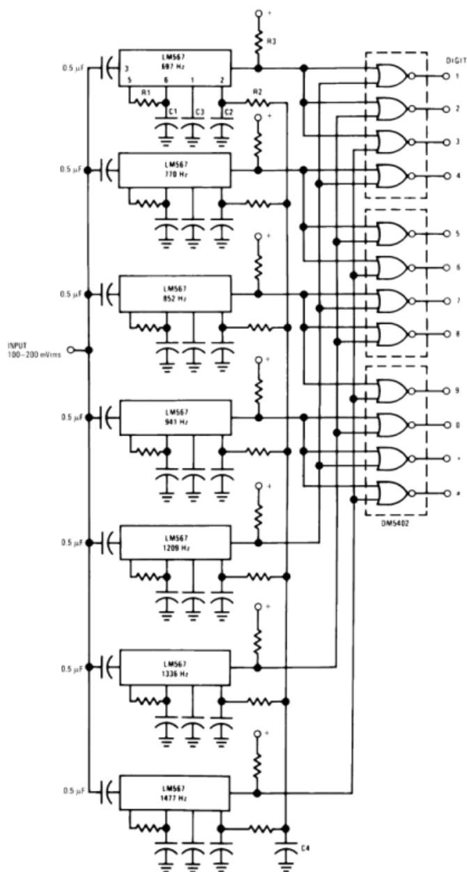
双音多频解码器
