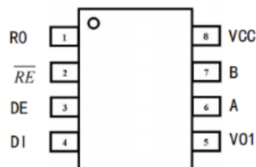
管脚配置
