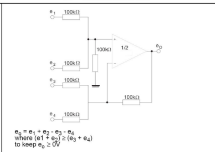
图4. 直流加法放大器
