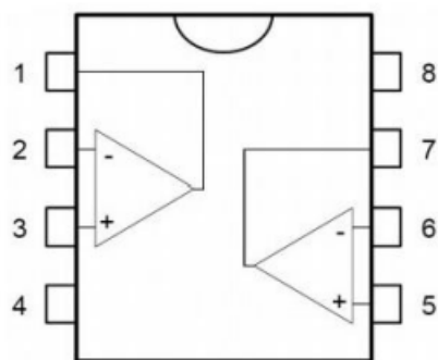
TL082(SOP8/DIP8)
