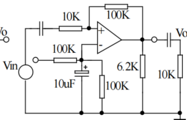
TL084 的其它应用
