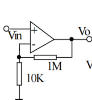
直流放大器
