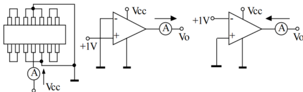
消耗电流 及输出电流 测试图
