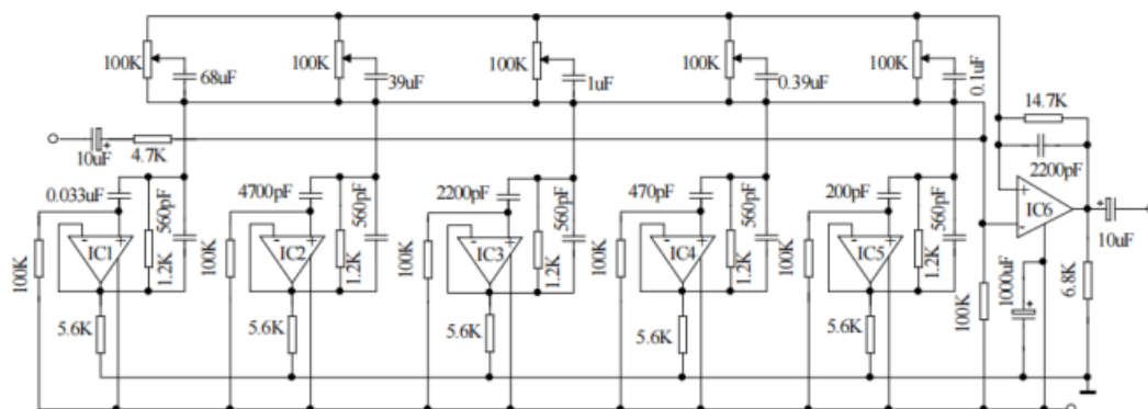
TL084 用于五频率音调控制电路
