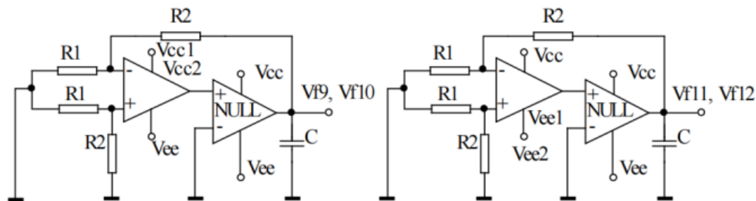
电源纹波抑制比 测试图
